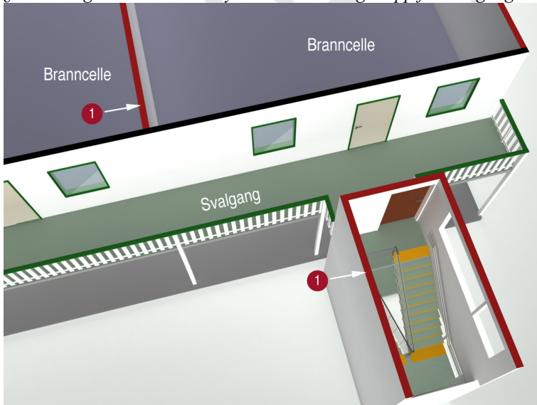
§ 11-14 Figur 5a: Brannbeskyttelse av rømningsstrapp fra svalgang.
