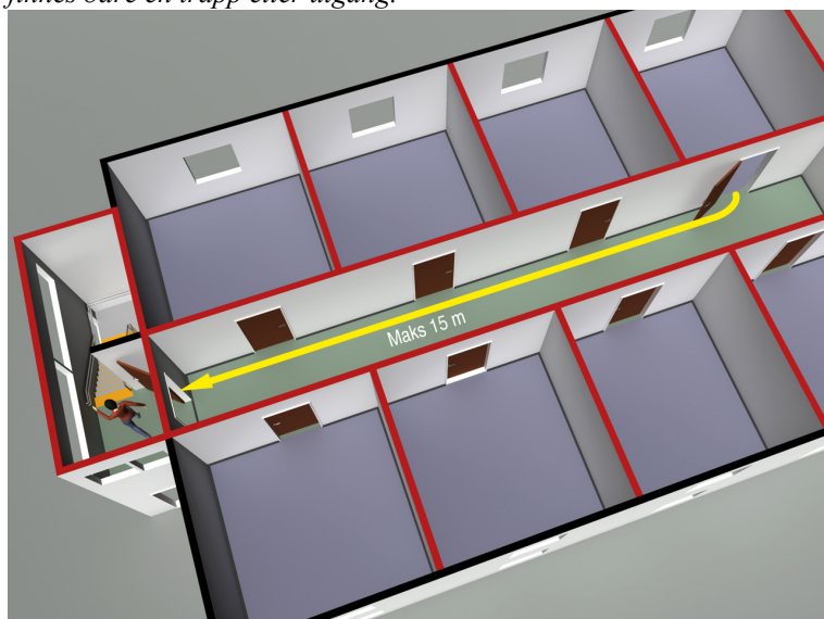
§ 11-14 Figur 2: Avstand fra dør i branncelle til nærmeste trapp eller utgang til sikkert sted må være maksimalt 15 m når det finnes bare én trapp eller utgang.
