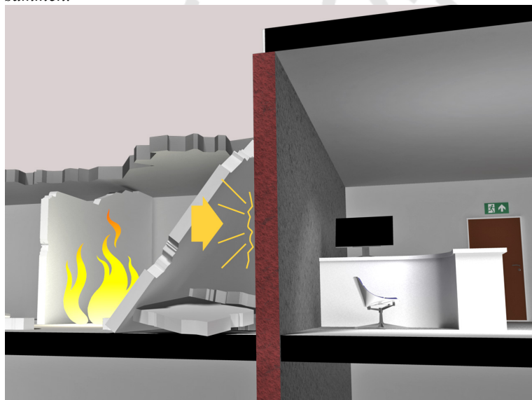
§ 11-6 Figur 2: Brannvegg må være stabil i forutsatt brannmotstandstid selv om byggverket på en eller begge sider faller sammen.
