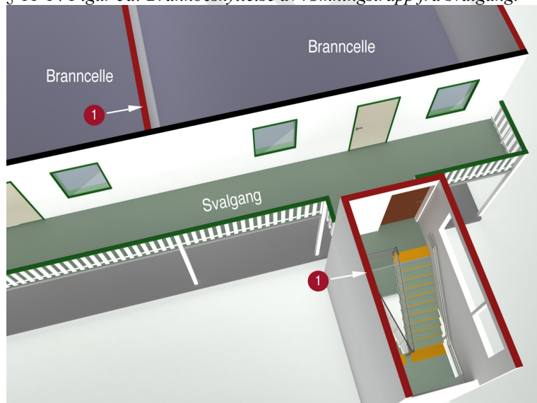
§ 11-14 Figur 5a: Brannbeskyttelse av rømningstrapp fra svalgang.
