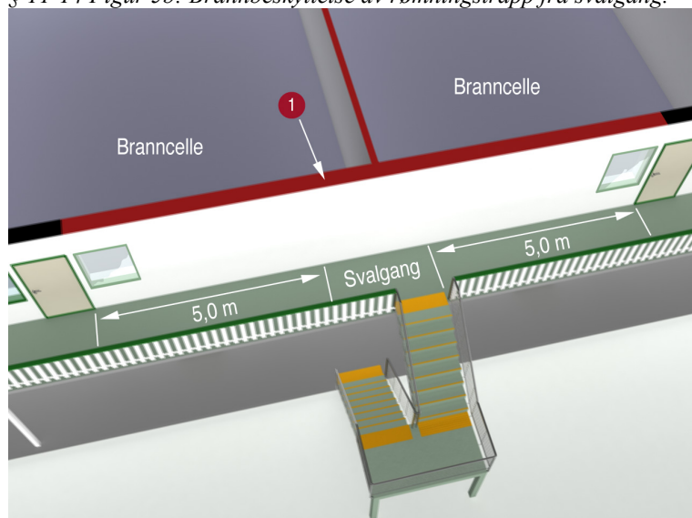
§ 11-14 Figur 5b: Brannbeskyttelse av rømningsstrapp fra svalgang.
