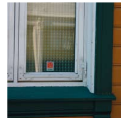
Nytt vindu (med feil glass) er plassert for dypt i den etterisolerte vegg.
