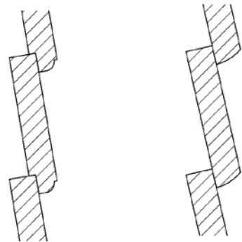
Enkeltfalset 1740-1850
