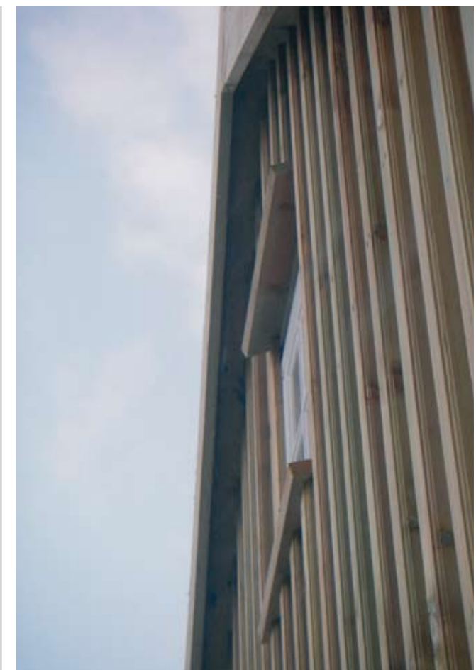
Eksempel på ny, høvlet tømmermannskledning med 28 mm profilert lekt/overbord. Ytre Sandgate 19, nybygg
