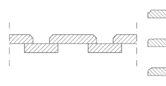
Tømmersmannskledning 1700-1850
