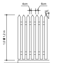
Eksempel på dimensjoner, stakitt
