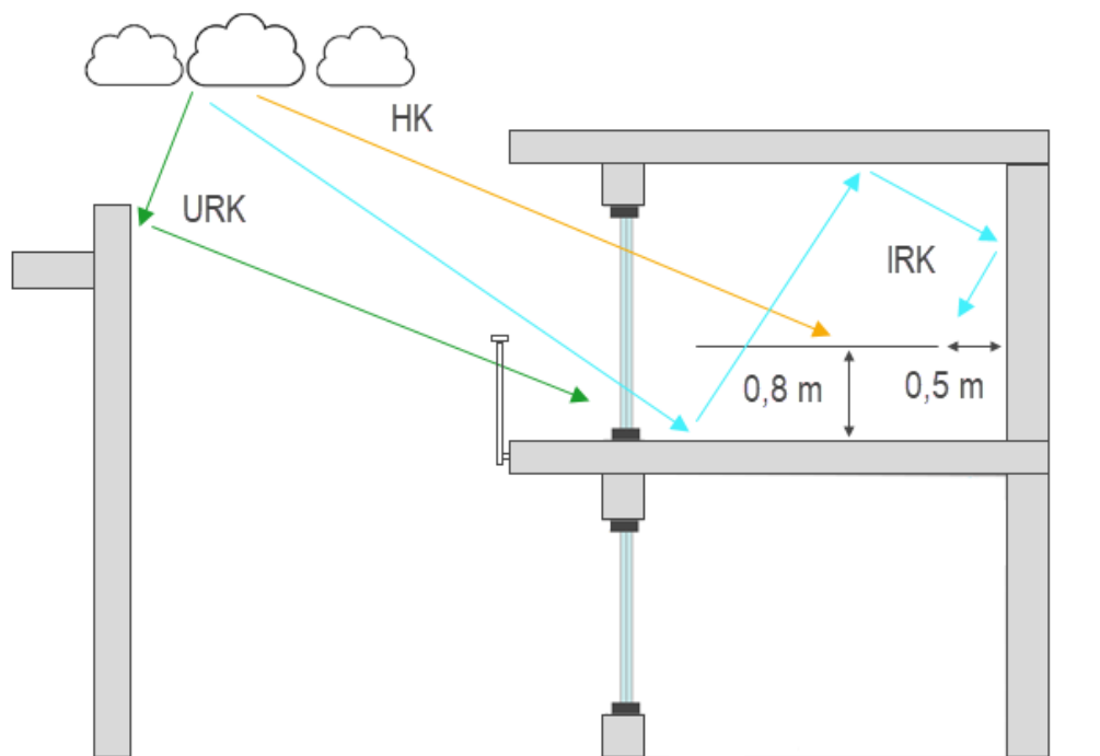
Figur 5: Komponentene som bidrar til dagslysfaktoren i et punkt og innvendig beregningsplan.
