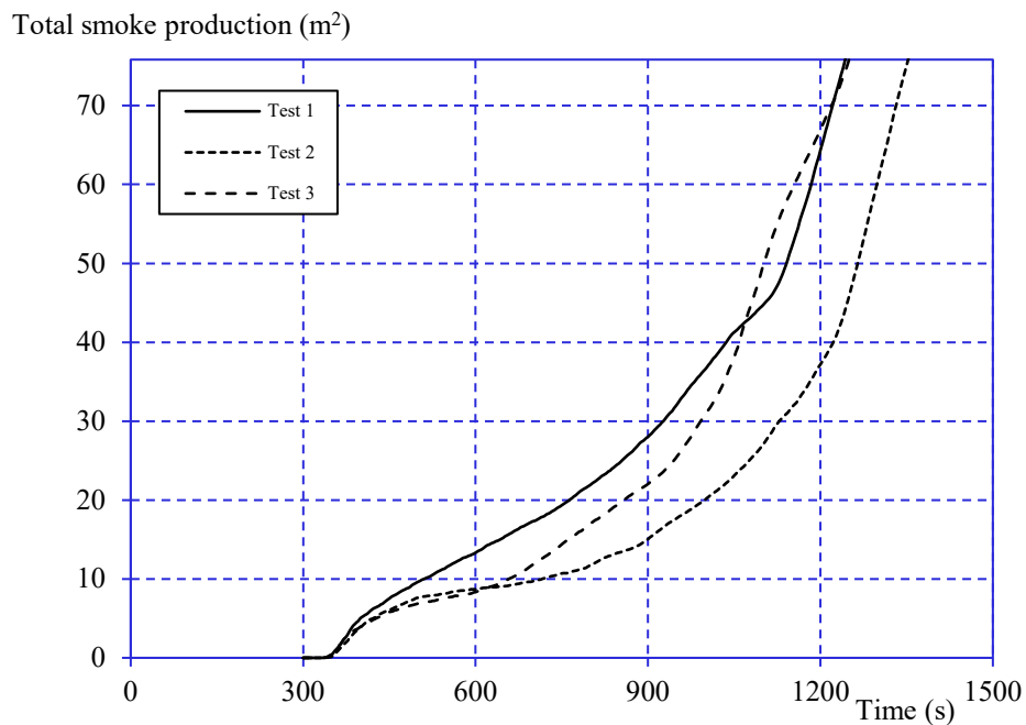
Diagram 4 Total rökproduktion (exklusive brännare).
