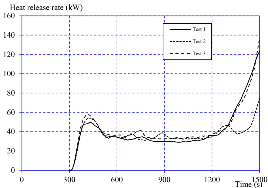
Diagram 1 Värmeutveckling (exklusive brännare), 30 sekunders medelvärde.
